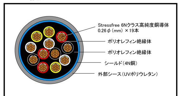
6N-DCP01 構造図
