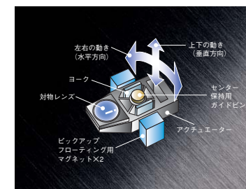
●軸摺動型ピックアップ構造図
