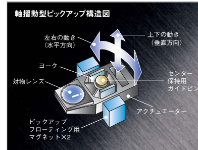
軸摺動型ピックアップ構造図
