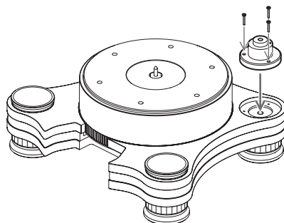
Vis de fixation de la tige de base du bras × 3
